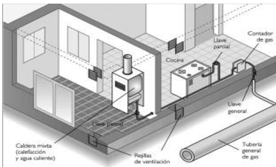
Esquema do enganche de gas natural a unha vivenda convencional
